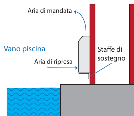
INSTALLAZIONE A PARETE
